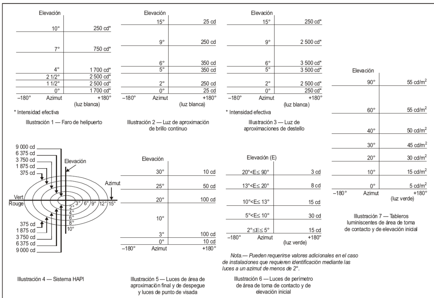
Figura 5-9H. Diagramas isocandela de las luces para las aproximaciones visuales y que no sean de precisión efectuadas con helicópteros
