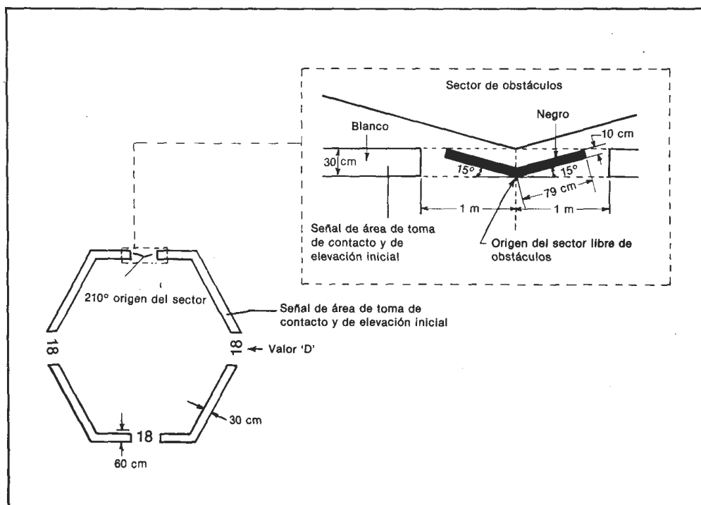
Figura 5-5H. Señal de sector despejado de obstáculos de heliplatforma
