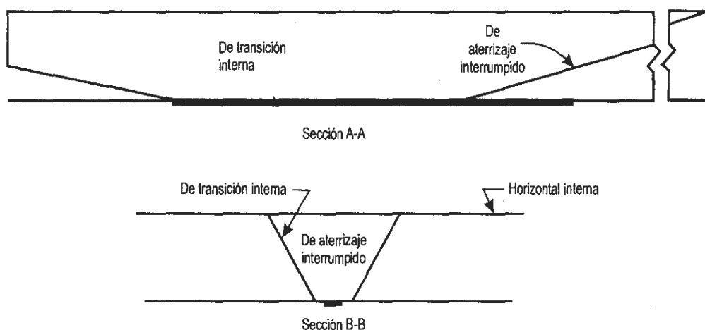
Continuación Figura 4.2. Superficies limitadoras de obstáculos de aproximación interna, de transición interna y de aterrizaje ininterrumpido
