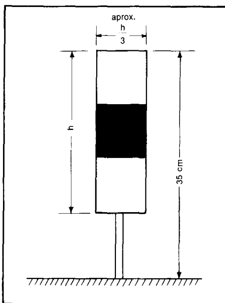
Figura 5-6H. Baliza de calle de rodaje aéreo
