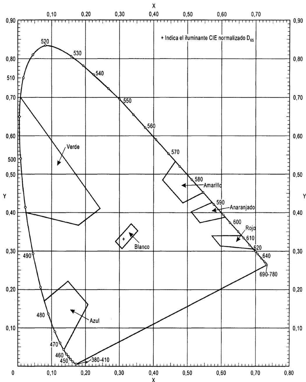
Figura A1 - 3. Colores de los materiales retrorreflektantes para las señales, letreros y tableros
