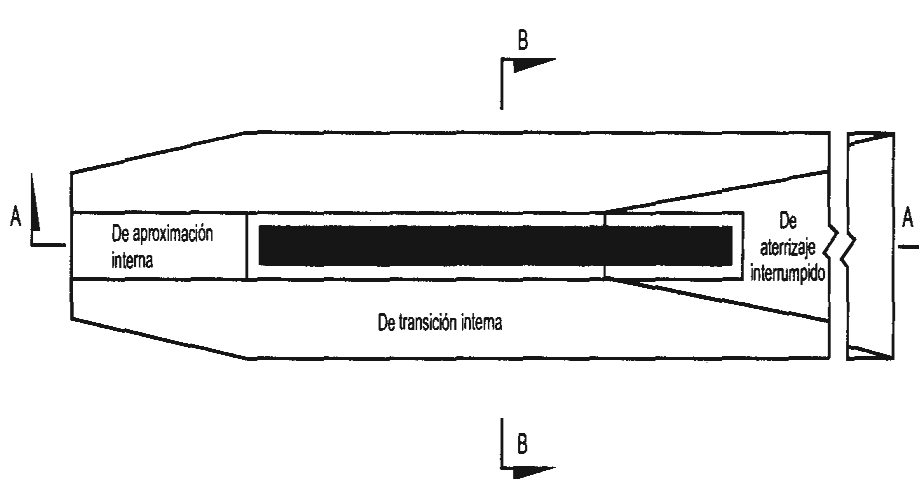
Figura 4.2. Superficies limitadoras de obstáculos de aproximación interna, de transición interna y de aterrizaje ininterrumpido
